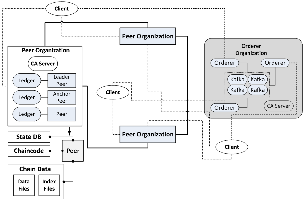
Hình 1: Các thành phần của mạng Hyperledger Fabric, mô hình kết nối giữa các peer và cấu trúc lưu trữ
