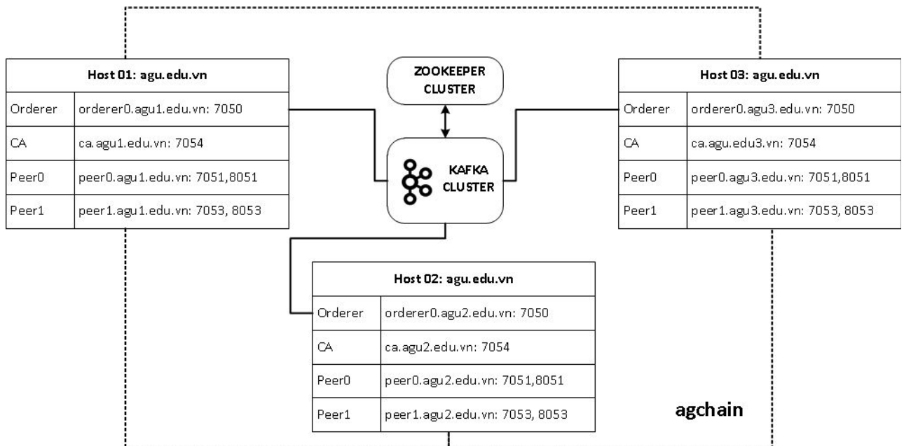
Hình 2: Mô hình kiến trúc mạng blockchain Hyperledger Fabric được đề xuất
